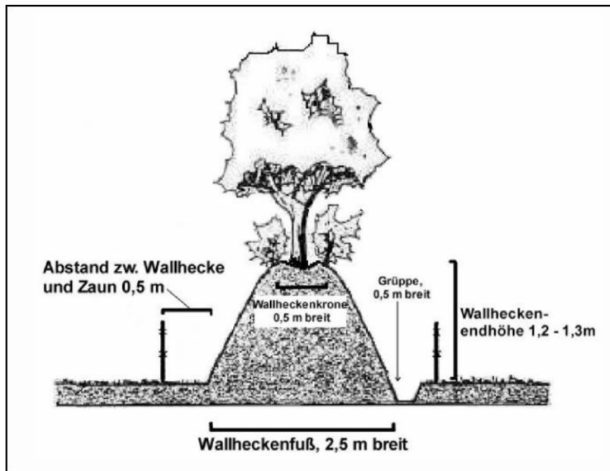
Aufbau und Querschnitt einer Wallhecke (schematisch).
