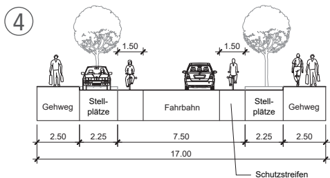
Schemaschnitte
